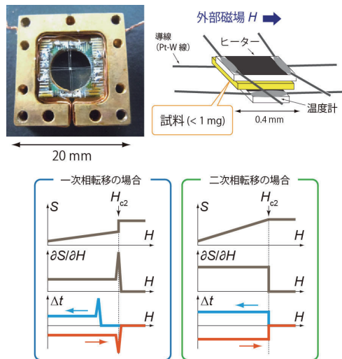
図 1：磁気熱量効果測定に実際に用いた熱量計。下段は一次相転移と二次相転移の場合の温度応答の比較。
