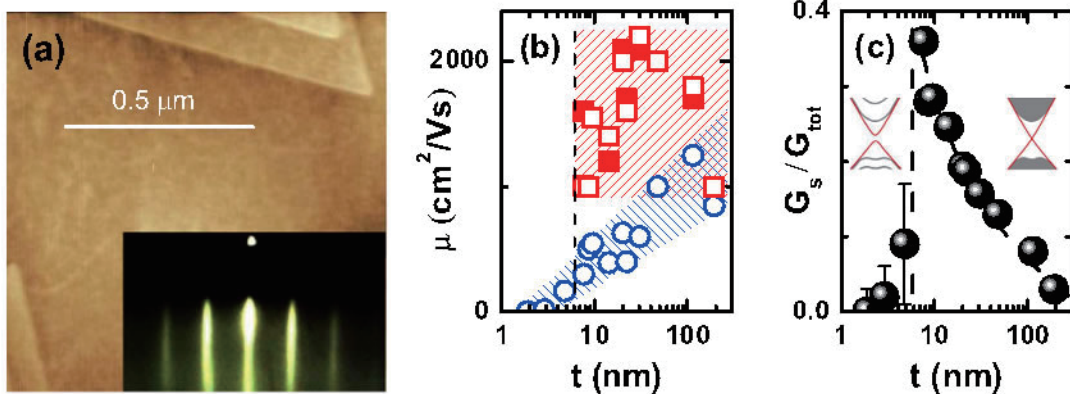
図2 : Bi 2 Se 3 薄膜の (a) AFM 像と RHEED 像、(b) 移動度と (c) 表面伝導度の膜厚依存性。
