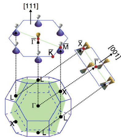
図 1: ARPES で決定した、(111) および (001) 表面におけるディラックコーン表面状態 [3]
