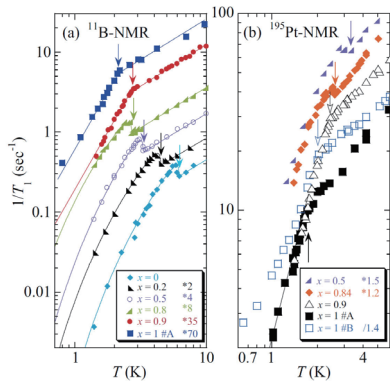
図 4 : \text{Li}_2(\text{Pt}_{1-x}\text{Pd}_x)_3\text{B} におけるスピン格子緩和率 1/T_1 の温度依存性。矢印は T_c を示す。
