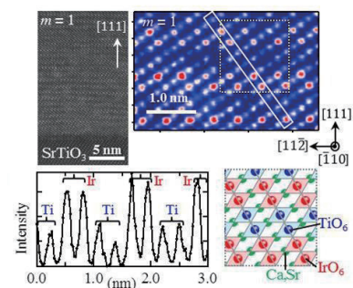
図 2 : 人工超格子 [(\text{Ca}_{0.5}\text{Sr}_{0.5}\text{IrO}_3)_2, (\text{SrTiO}_3)_2] の断面透過電子顕微鏡 (高角散乱環状暗視野モード)。
