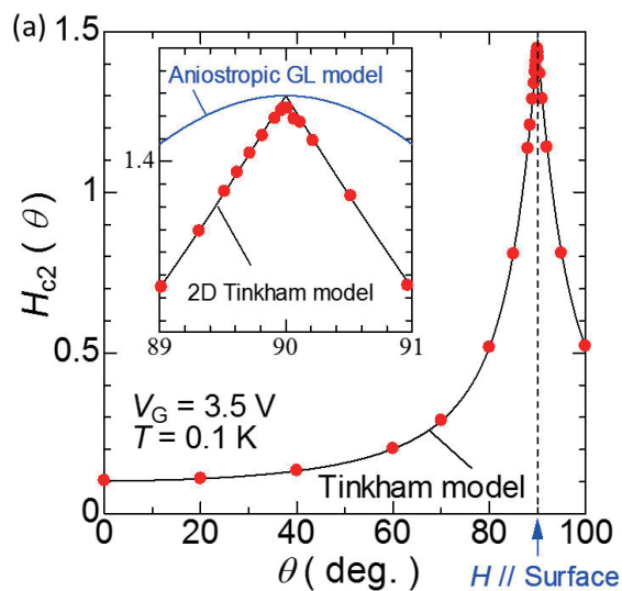
図 1 : SrTiO 3 電気二重層トランジスタにおける電場誘起超伝導の上部臨界磁場の方位依存性
