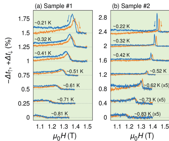
図 2：磁気熱量効果測定実験 [1] で得られた試料の相対温度 \Delta t 。見やすいように、データを縦にずらしている。また、上げスweepのデータに関しては \Delta t に -1 をかけて符号を正にしている。(b) の Sample #2 が本文中で言うところの「神サンプル」である。
