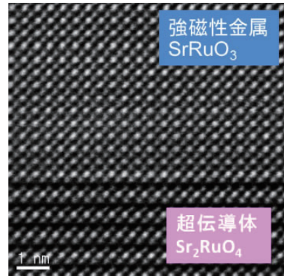
図2: \text{Sr}_2\text{RuO}_4 単結晶の上に強磁性金属 \text{SrRuO}_3 薄膜をエピタキシャル成長させた系の模式図と透過型電子顕微鏡写真 [7]。スケールバーは 1 ナノメートル。
