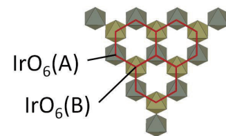
図 1 : (111) 方向に積層した人工超格子 [(\text{SrIrO}_3)_2, (\text{SrTiO}_3)_2] の模式図。
