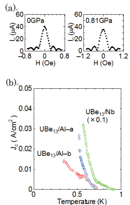
図 1 (a) UPt_3 と Al の間のジョセフソン臨界電流の磁場依存性と (b) UBe_{13} のジョセフソン臨界電流の温度依存性。
