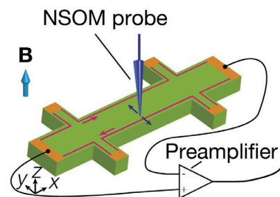
図 1 : 円偏光近接場走査型光学顕微鏡を用いたスピン分裂量子ホール系カイラルエッジ状態の空間マッピング測定方法の概略図。
