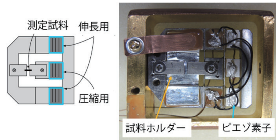
図1：ピエゾ素子を用いた試料伸縮装置。
