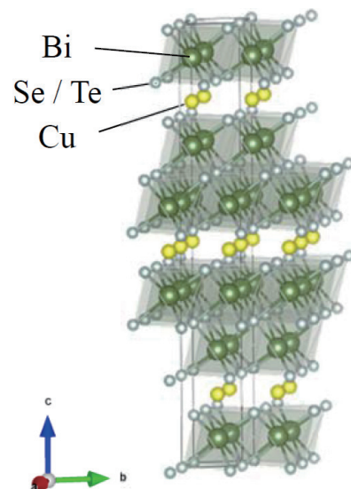
図 1 : \text{Cu}_{0.25}\text{Bi}_2(\text{Te}_x\text{Se}_{1-x})_3 の結晶構造
