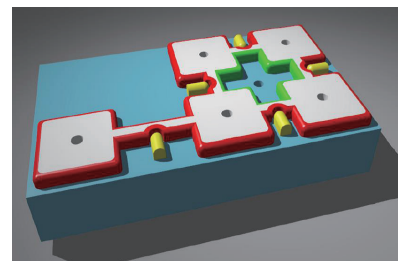
図 1 : マヨラナ量子ビットの NOT ゲートの模式図
