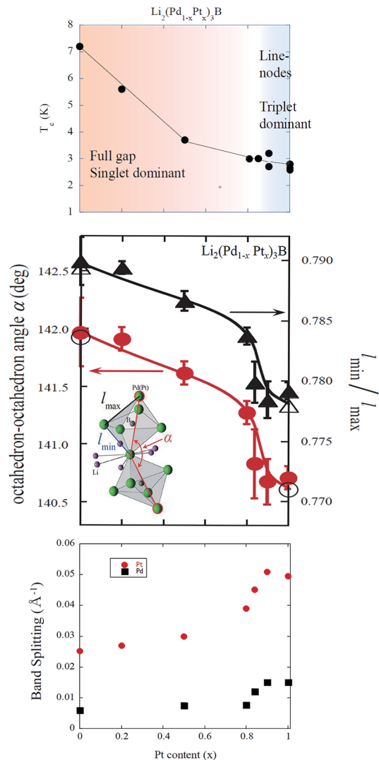
図 6 : (上) 超伝導対称性の変遷を模式的に描いた。(中) 反転対称性の破れの度合いが Pt 組成量とともに変化する様子。(下) R 点におけるバンド分裂の様子。
