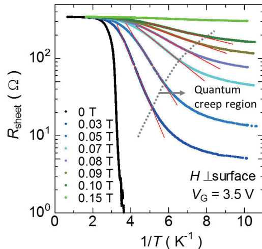
図 2: 量子磁クリープ現象を示す SrTiO 3 電気二重層トランジスタ面垂直磁場中における面抵抗の温度依存性 (アレニウスプロット)。
