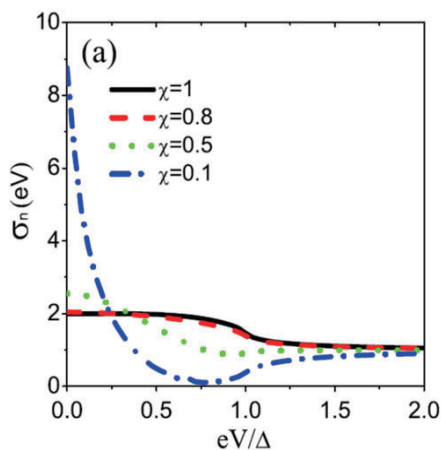
図5：様々な透過率 \chi におけるコンダクタンス
