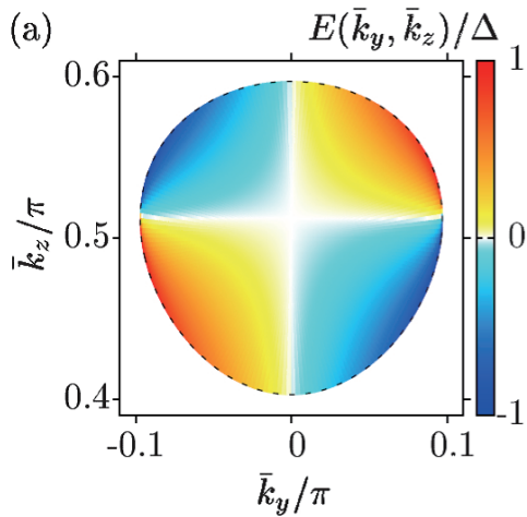
図1：ワイル半金属のBCS状態における(a) Andreev束縛状態のエネルギー分散
