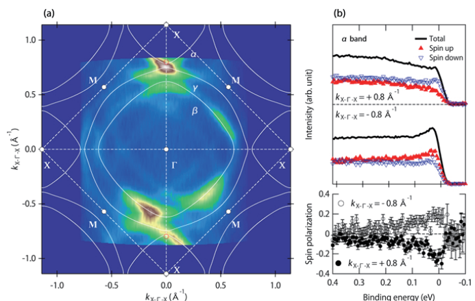
図 2 : \text{Sr}_2\text{RuO}_4 におけるスピン分解 ARPES データ
