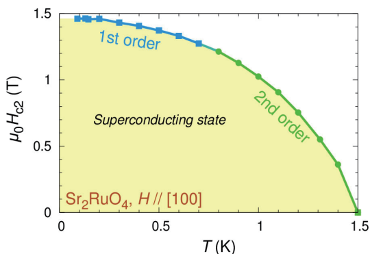
図3：比熱測定 [2] から得られた \text{Sr}_2\text{RuO}_4 の H // [100] での超伝導相図。水色の四角は H_{c2} での転移が一次相転移になっていることを示す。
