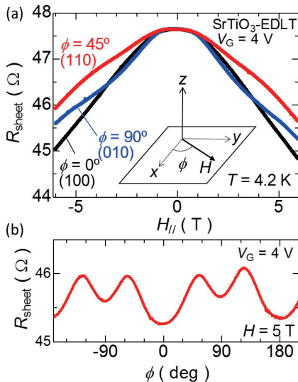
図 1: 電気二重層トランジスタにより高電子密度を誘起した SrTiO 3 表面における電気抵抗の (a) 面内磁場依存性、(b) 面内磁場方位依存性。
