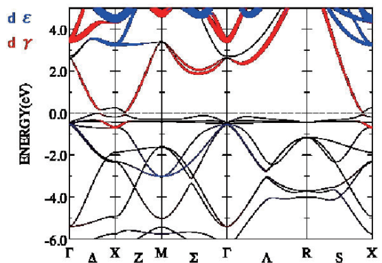
図5： \text{SmB}_6 のバンド構造
