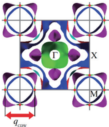
図 1: \text{LaPt}_2\text{Ge}_2 のフェルミ面
