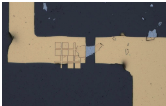
図1：試作したデバイスの写真（トポロジカル絶縁体の剥離薄膜試料の両端に Au 電極をつけた。試料サイズは数ミクロン程度。）
