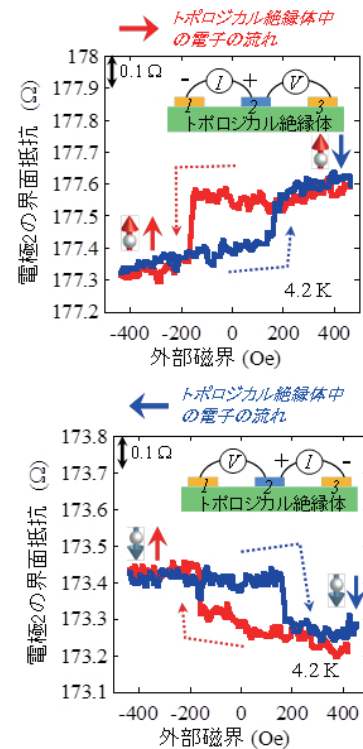
図：(上) \text{Bi}_{1.5}\text{Sb}_{0.5}\text{Te}_{1.7}\text{Se}_{1.3} を用いたスピンデバイスにおける磁気抵抗効果の測定結果および(下)電流の向きを反転した場合の測定結果、矩形信号がトポロジカル絶縁体のスピン流に起因。
