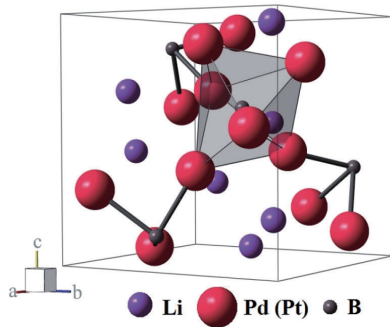
図 3 : \text{Li}_2(\text{Pt}_{1-x}\text{Pd}_x)_3\text{B} の結晶構造
