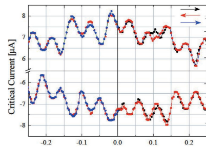
図1：ハイブリッドSQUIDの超伝導臨界電流の磁場干渉パターン。半分の量子磁束に対応する周期も観測。
