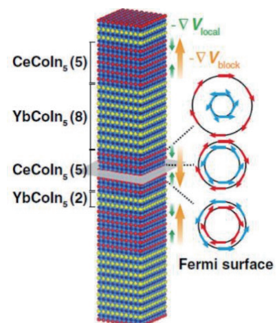
図 1: 重い電子系超伝導体 \text{CeCoIn}_5 と、同じ結晶構造を持つ通常金属 \text{YbCoIn}_5 の超格子構造。YbCoIn 5 の厚みに変調をかけることで空間反転対称性の破れの度合いを制御できる。
