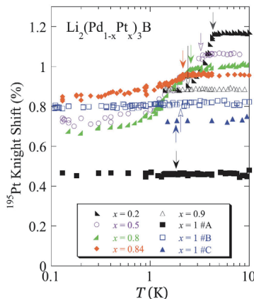
図 5 : \text{Li}_2(\text{Pt}_{1-x}\text{Pd}_x)_3\text{B} におけるナイトシフトの温度依存性。矢印は T_c を示す。
