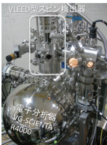
図 1 : VLEED 型スピン分解 ARPES 装置
