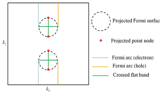
図2：ワイル半金属BCS状態に現れるゼロエネルギー状態
