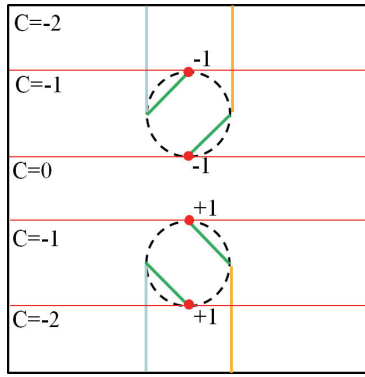
図4：チャーン数から期待されるゼロエネルギー Andreev 束縛状態
