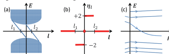
図1: カイラル d 波超流動体の全軌道角運動量とスペクトラルフロー。
