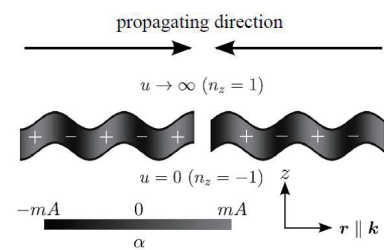
図 1 : ドメイン壁を伝わる南部ゴールドストーン励起。壁の振動と共に、位相の振動も励起される。
