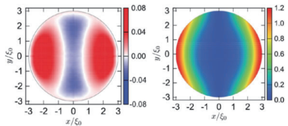
図3: スピン三重項 p 波超伝導体の微小円板に発現する奇周波数超伝導状態の計算結果 [8]。左: 局所磁化率は図で左右の端で正となる。右: 正の磁化率に対応する部分で奇周波数 s 波状態が生じている。
