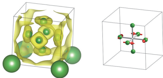
図6： \text{SmB}_6 の伝導バンドの波動関数の空間分布（左）と T_{2g} フォノンモード（右）
