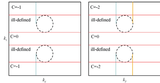
図3：ワイル半金属相におけるチャーン数(左)及びBdG形式におけるチャーン数(右)
