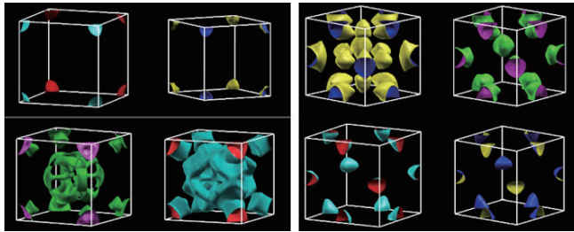
図7: \text{Li}_2(\text{Pt}_{1-x}\text{Pd}_x)_3\text{B} のフェルミ面。4部分から構成されており、それぞれが反対称軌道相互作用によって分裂している。
