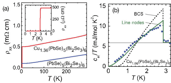
図3：新超伝導体 \text{Cu}_x(\text{PbSe})_5(\text{Bi}_2\text{Se}_3)_6 の (a) 電気抵抗率、(b) 電子比熱の温度依存性
